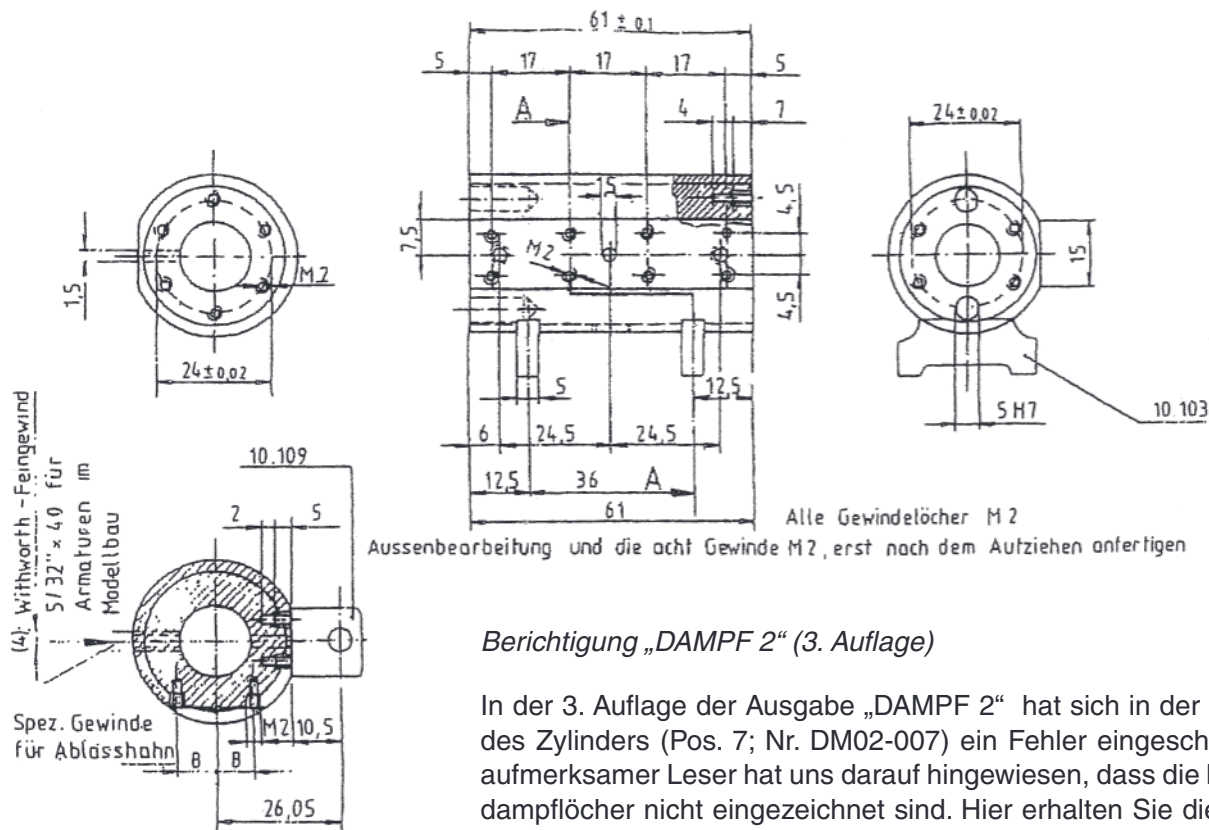
Schnitt A-A
